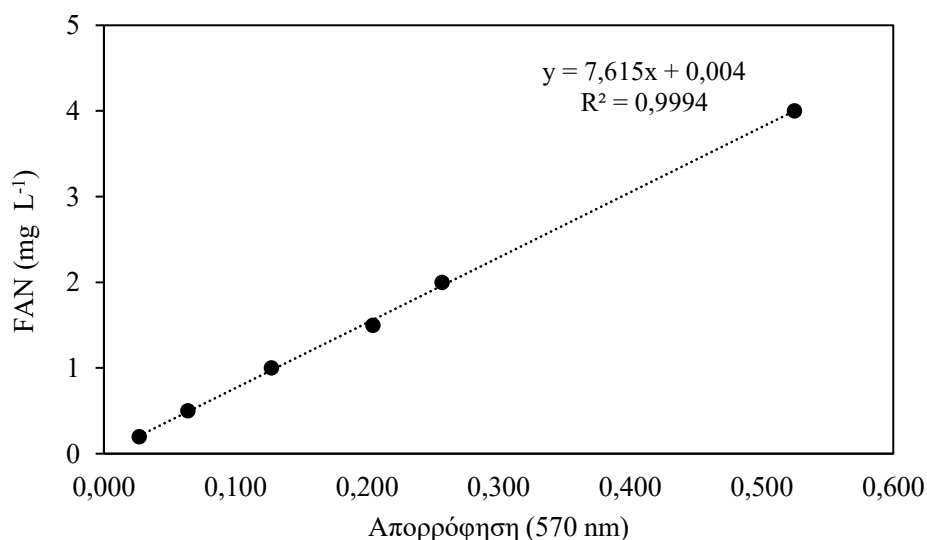
Διάγραμμα 3.2: Πρότυπη καμπύλη γλυκίνης για τη μέθοδο FAN
