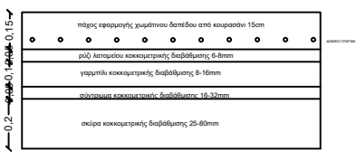
ΛΕΠΤΟΜΕΡΕΙΑ ΧΩΜΑΤΙΝΟΥ ΔΑΠΕΔΟΥ
