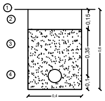
ΛΕΠΤΟΜΕΡΕΙΑ ΧΑΝΤΑΚΙΟΥ ΚΑΛΩΔΙΩΝ
